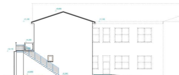
POHLED JIŽNÍ
